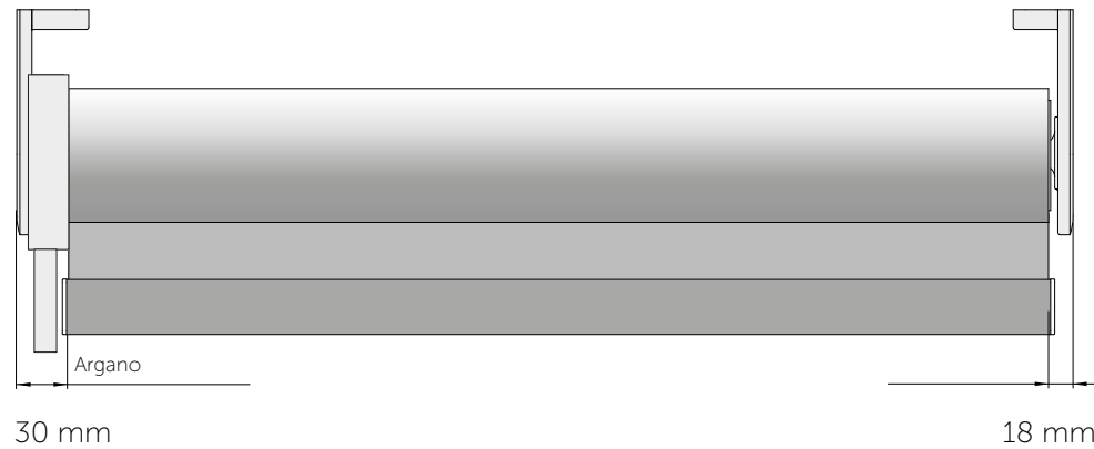
STAFFA E ARGANO
